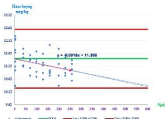
Hình 4. Đồ thị biểu thị hạn sử dụng của Arsenic Hình 5. Đồ thị biểu thị hạn sử dụng của Thủy ngân
