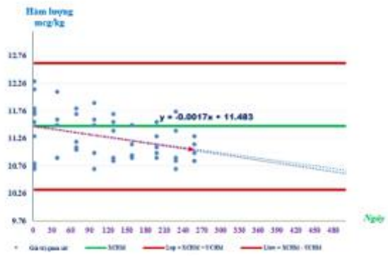
Hình 3. Đồ thị biểu thị hạn sử dụng của cadmi
