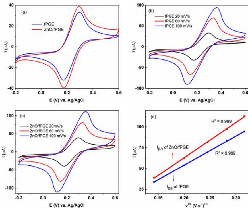
Hình 5. Đường cong CV (a) fPGE, ZnO/fPGE trong dung dịch [(Fe(CN)_6]^{3-/4-} 5mM /M KCl 0,1 với tốc độ quét of 20 mV/s ; (b, c) CV của fPGE and ZnO/fPGE ở tốc độ quét khác nhau (20, 60, 100 mV/s), và (d) đồ thị của I_{pa} - v^{1/2}
